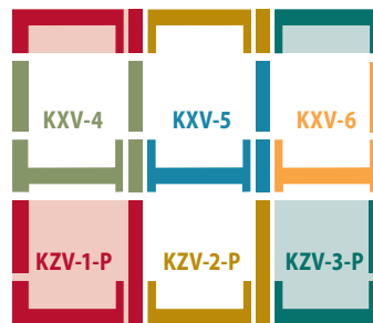
Блочне сполучення B3/2
